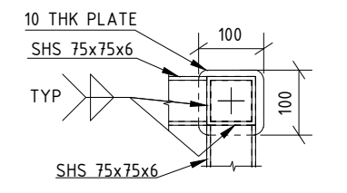
DETAIL -2 TYP (SCALE 1:10)
