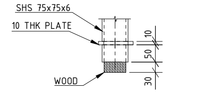
DETAIL -1 TYP (SCALE 1:10)
