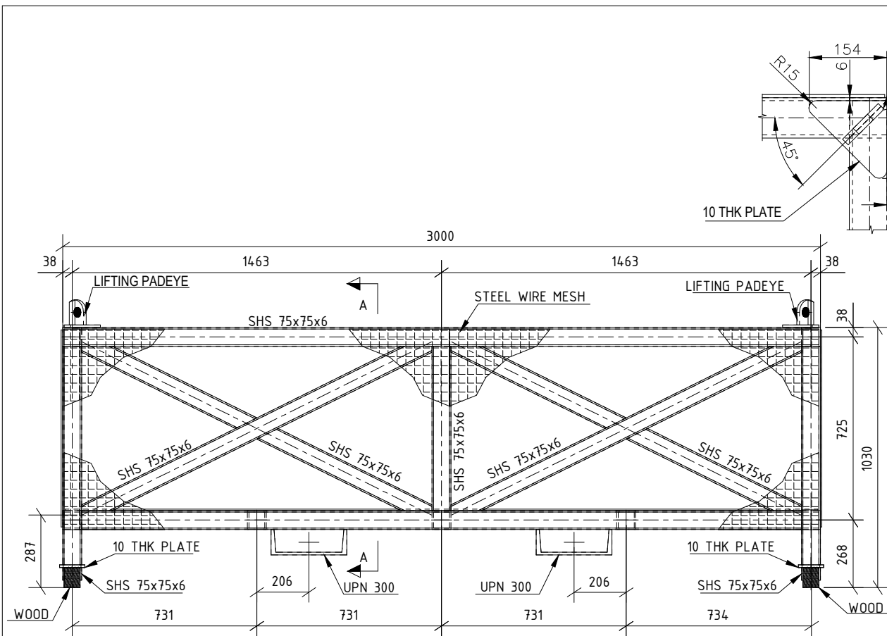
LIFTING BASKET (3.0 MT S.W.L.) FRONT EL VIEW (SCALE 1:20)
